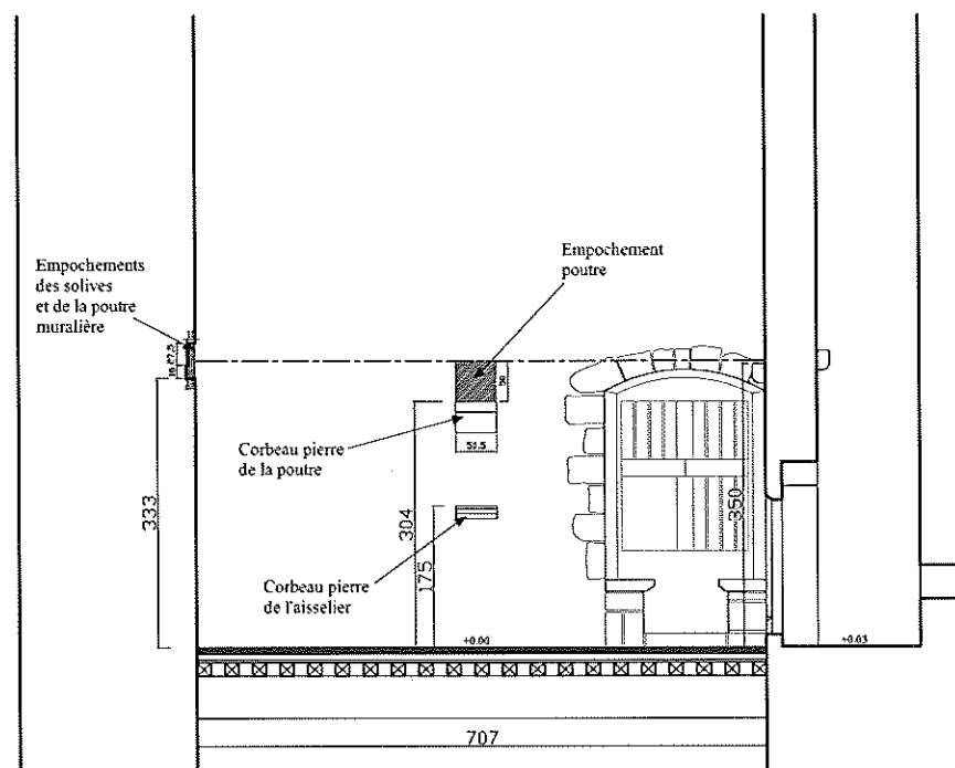
ELEVATION NORD
