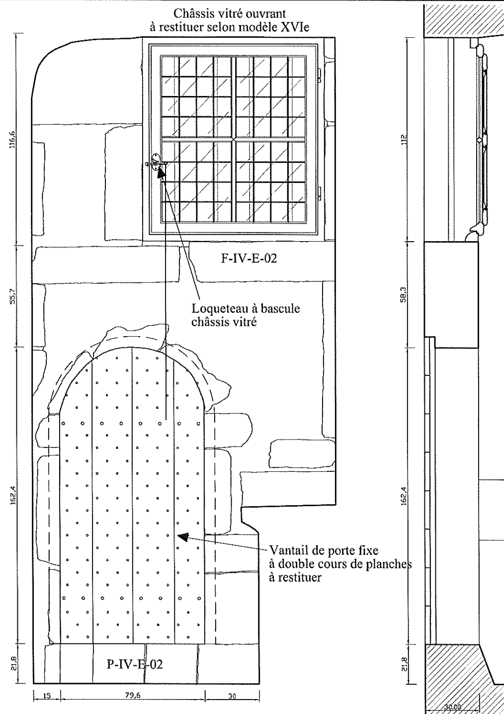
Elévation intérieure originelle de la baie Est Elévation intérieure après transformation Restitutions dessinées par J-M Paoli, octobre 1997
