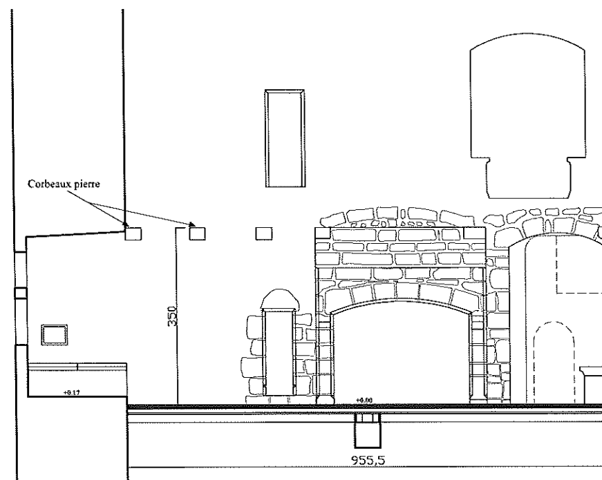
ELEVATION EST
