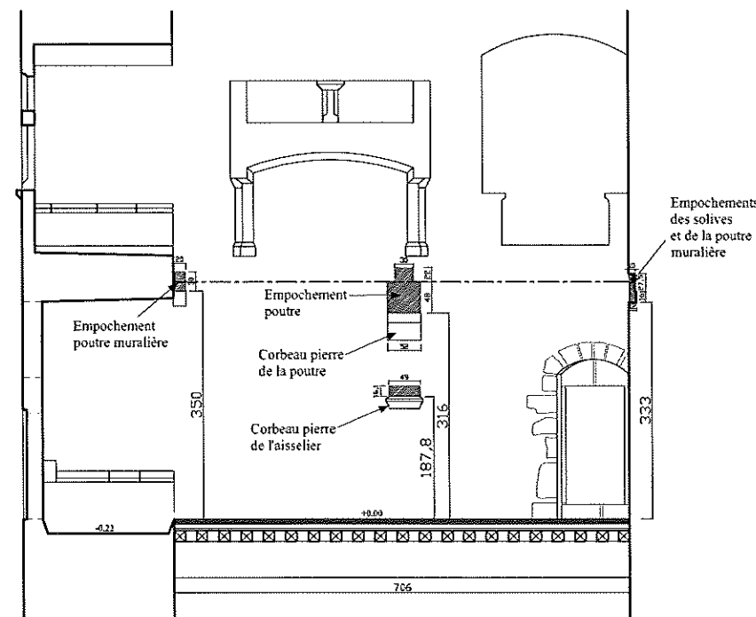
ELEVATION SUD
