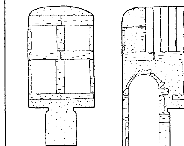
Elévation intérieure originelle de la baie Est Elévation intérieure après transformation Restitutions dessinées par J-M Paoli, octobre 1997
